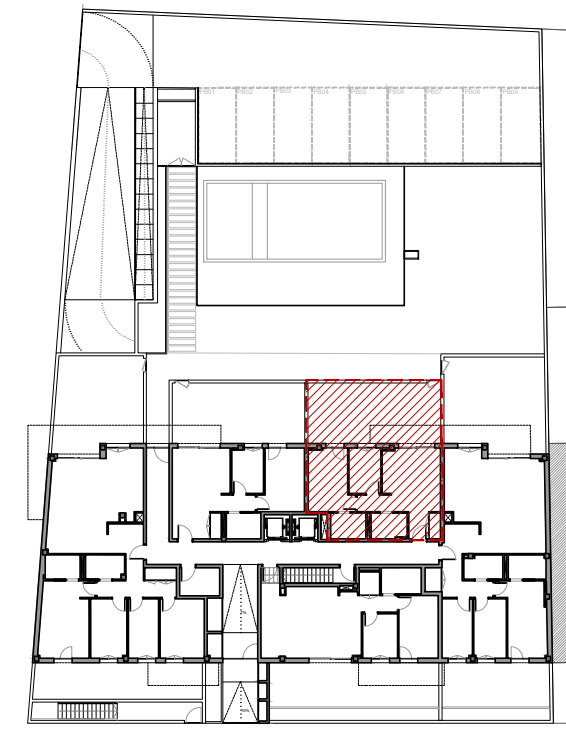
PLANTA BAIXA
